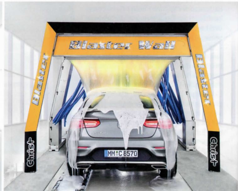
Der Foam Wall ist als Anbau-Option für den Alu-Premium-Bogen erhältlich
